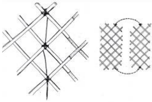
شکل ۵ - طرز اتصال دو تارم به یکدیگر
