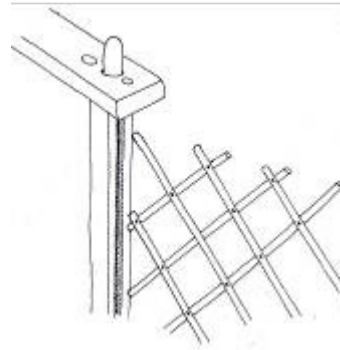
شکل ۴ - جزئیات اتصال تارم با چهارچوب در ورودی
