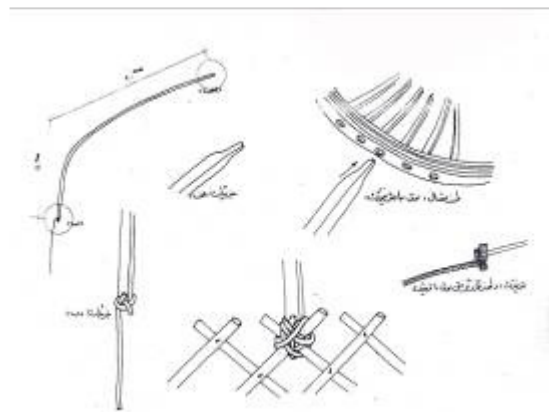
شکل ۸- جزییات اتصال « اوق » با تارم و « توینوک »
