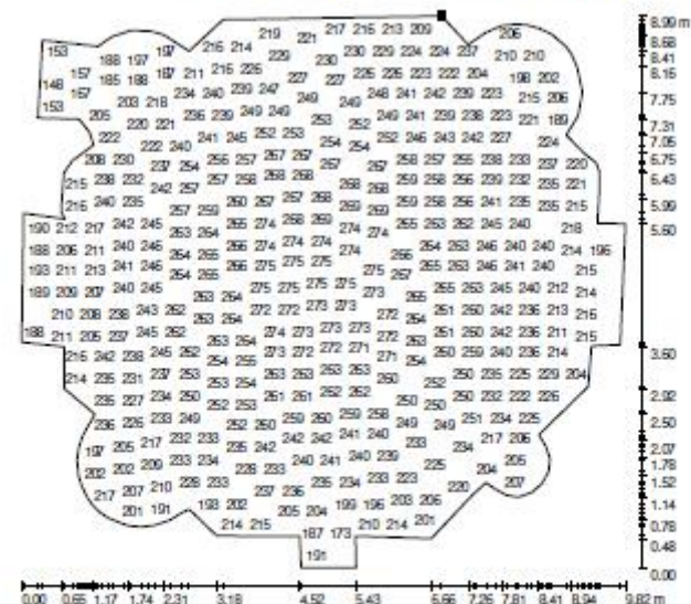
Cupola lampadine + S-line5630 / Pavimento / Grafica dei valori (E)
